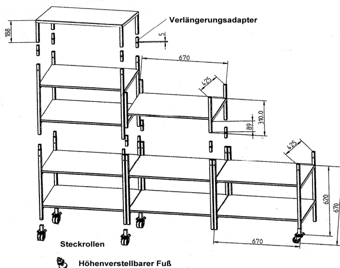
Gerätekonsole
